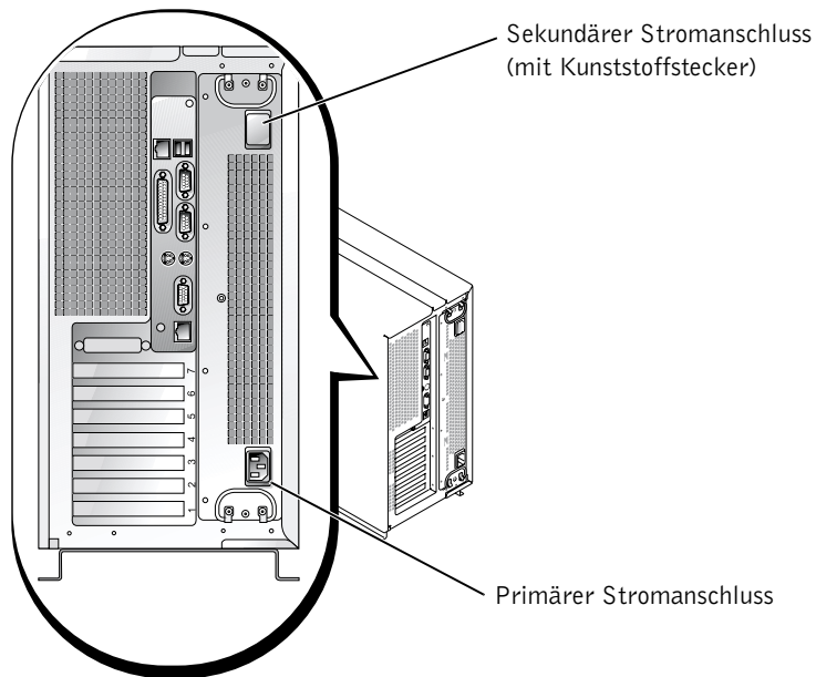
Abbildung 4-2. Stromanschlüsse
